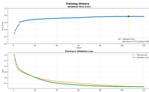
(α') UNETR
