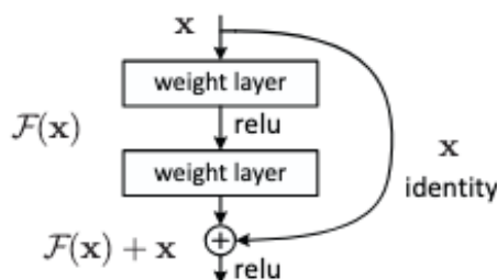
Σχήμα 4.2: Μηχανισμός residual connection στην αρχιτεκτονική ResNet [1]
